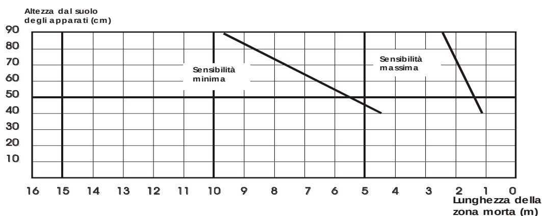
Figura 6 - Lunghezza della zona morta in prossimità degli apparati in funzione dell'altezza dal centro degli stessi al suolo per ERMO 482/. 80-120-200
