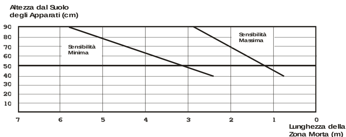
Figura 5 - Lunghezza della zona morta in prossimità degli apparati in funzione dell'altezza dal centro degli stessi al suolo per ERMO 482/. 50
