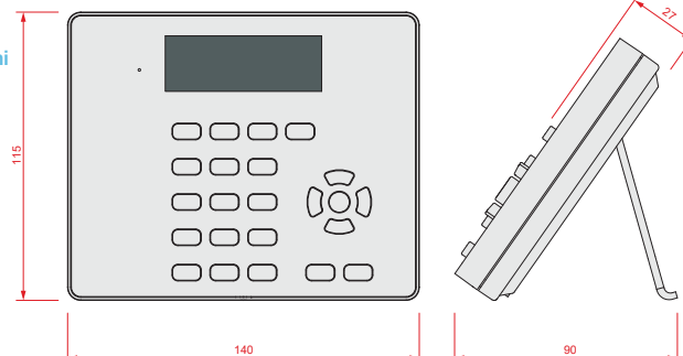
Aria/HG - dimensioni
