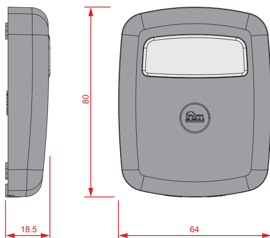
nBy/S - dimensioni
