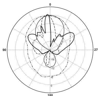
Curva verticale
