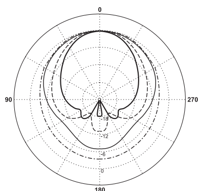
Curva orizzontale
